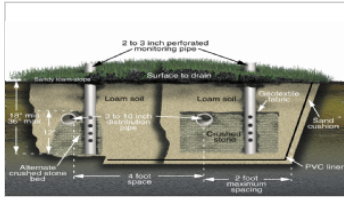
Evapotranspiration bed STA
