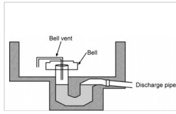
Siphon
